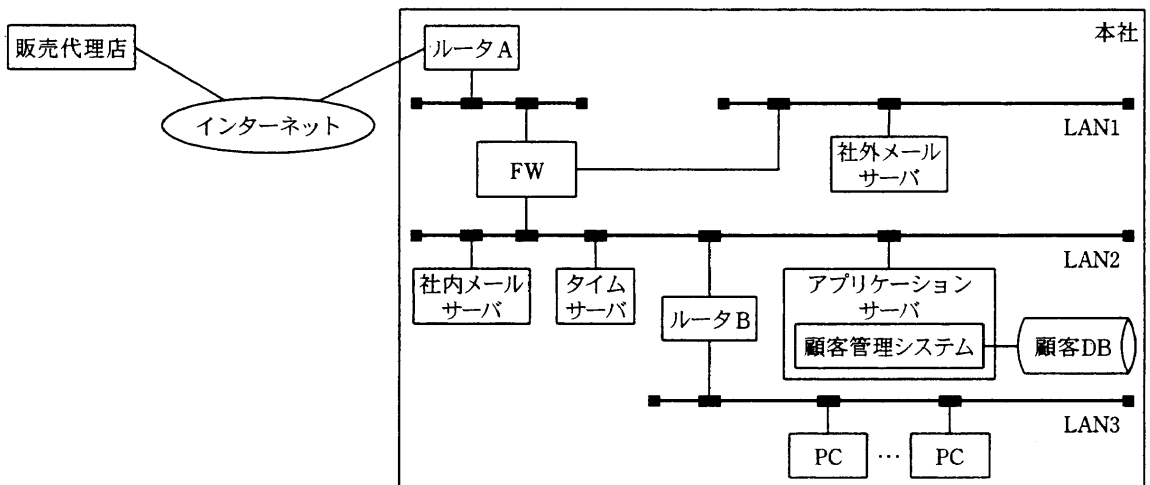
図 M 社のシステム構成
