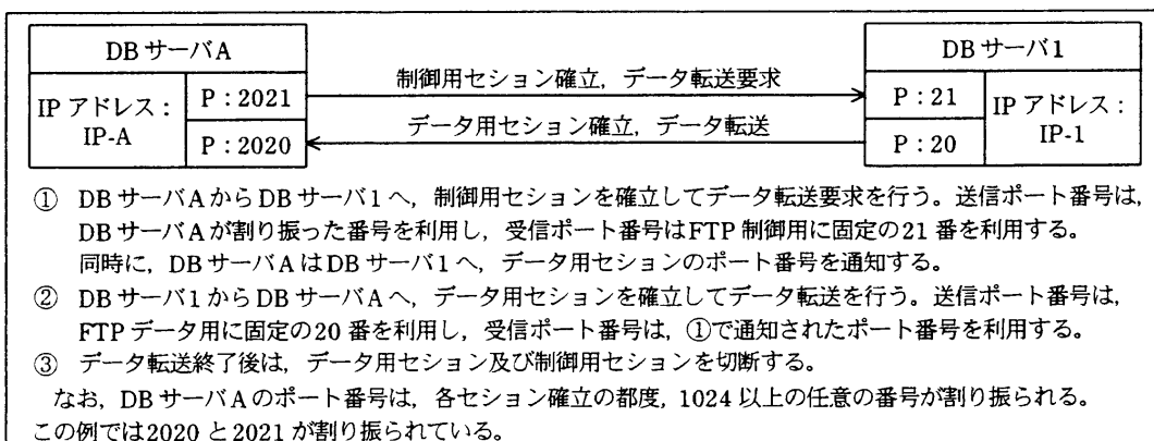
図 2 K 社におけるデータ転送手順と転送例
