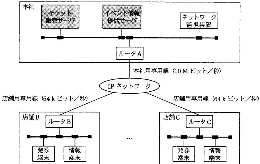
図 1 T 社のチケット販売システムの構成
