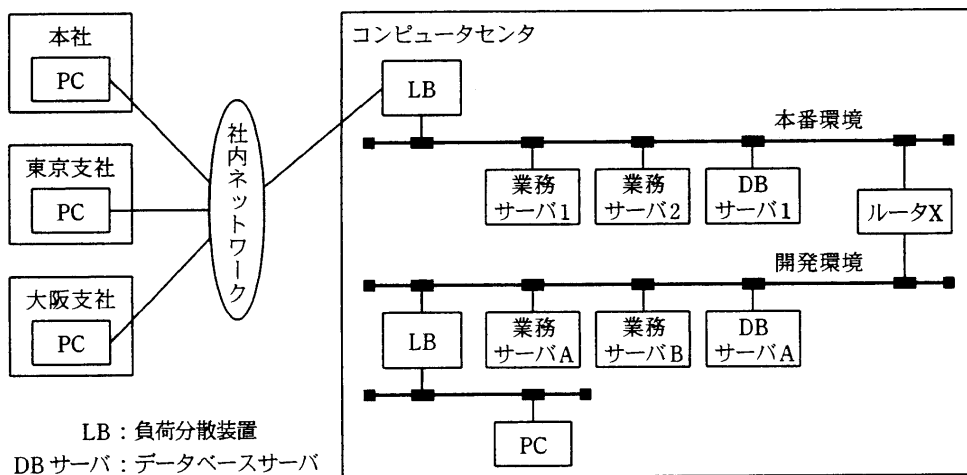
図1 受注管理システムの構成
